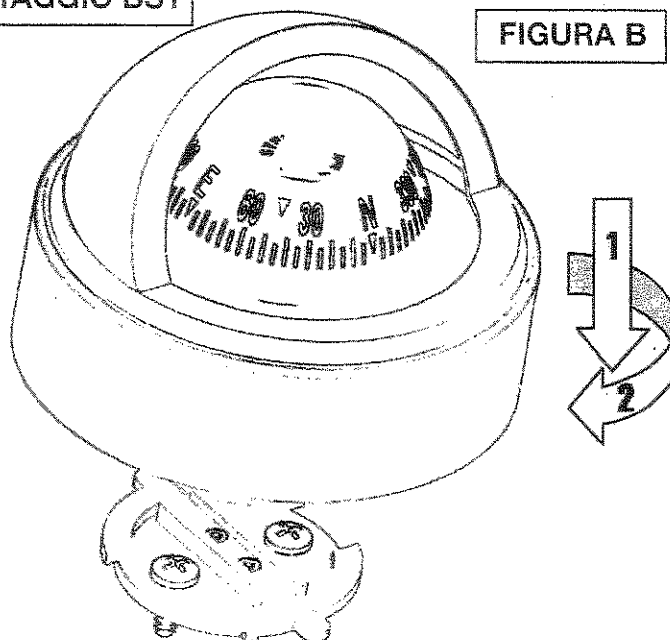
SCHEMA DI MONTAGGIO BS1
