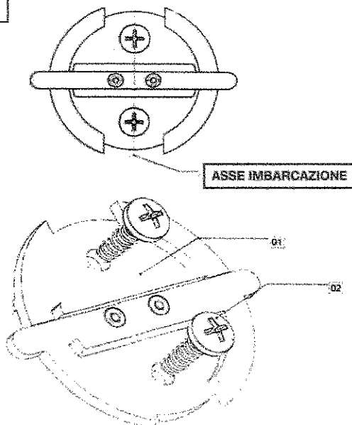
SCHEMA DI MONTAGGIO BS1
